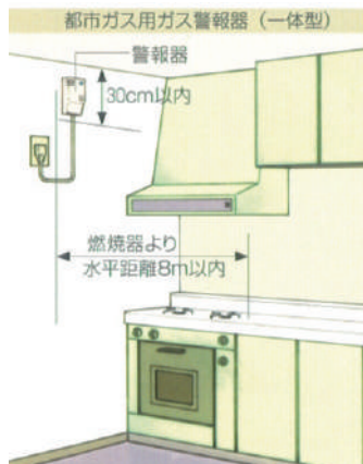
ガス警報器設置位置 (* ガスの種類で設置場所が異なります)
